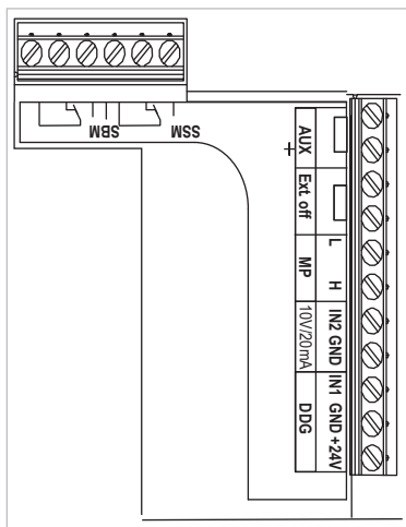
Fig. 27: Styrplintar
