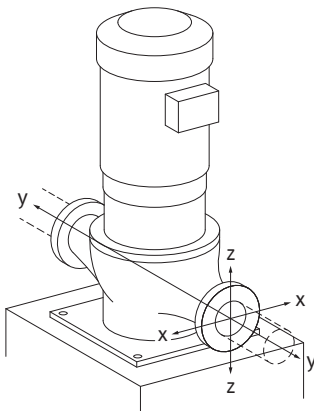
Kuva 23: Kuormitustapaus 17A
