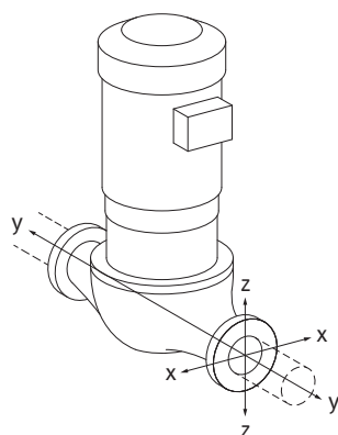
Rys. 22: Przewidywany przypadek obciążenia 16A
