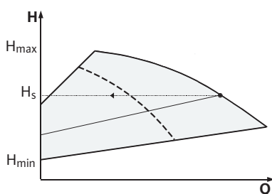
Rys. 15: Regulacja \Delta p -v (praca równoległa)
