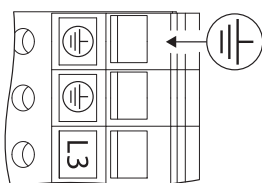
Rys. 29: Dodatkowe uziemienie
