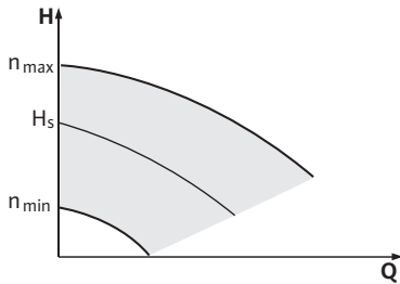
Рис. 12: Режим управления
