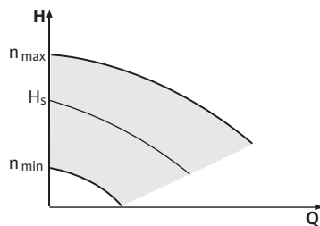
Kuva 46: Säädinkäyttö
