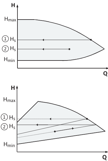
Рис. 45: Регулирование Δp-c/Δp-v
