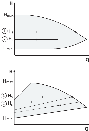
Kuva 45: Säätö \Delta p-c/\Delta p-v
