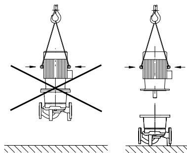
Kuva 20: Moottorin kuljetus
