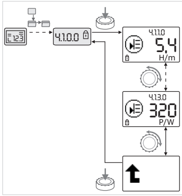
Kuva 42: Tietojen hakeminen näyttöön
