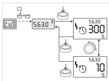
Рис. 40: Настройка с возвратом к элементу меню «Выбор/настройка»
