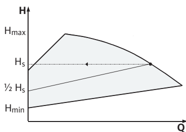
Rys. 11: Regulacja Δp-v
