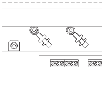
Rys. 26: Ekranowanie przewodu
