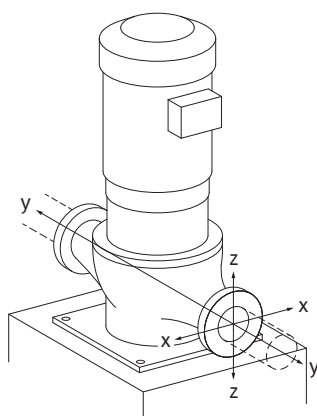
Fig. 23: Расчетный случай нагрузки 17A
