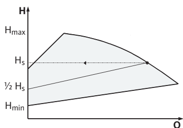
Рис. 11: Регулирование Др-в
