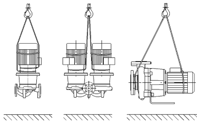
Рис. 7: Транспортировка насоса
