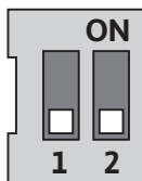
Fig. 31: DIP-brytare
