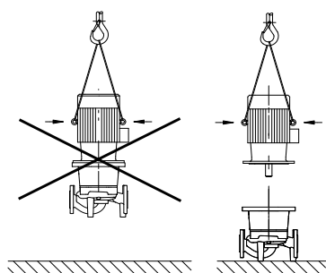
Kuva 8: Moottorin kuljetus
