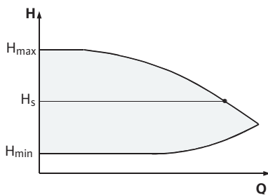
Rys. 10: Regulacja Δp-c
