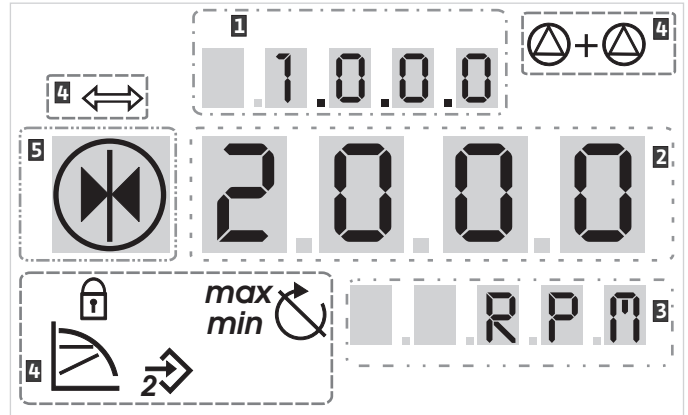
Kuva 32: Näytön rakenne
