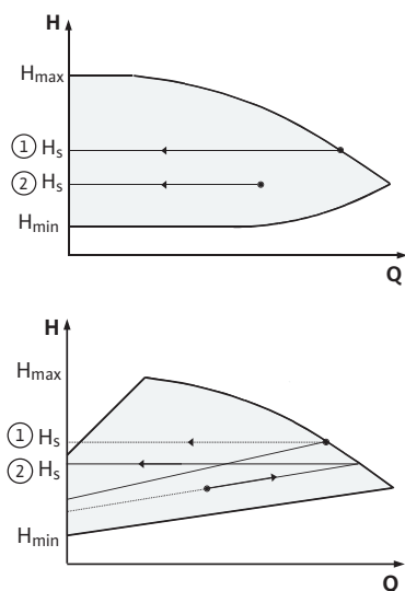
Rys. 45: Regulacja \Delta p\text{-}c/\Delta p\text{-}v
