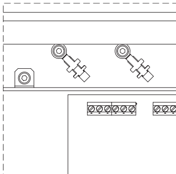
Kuva 26: Kaapelin suojaus
