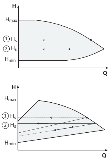
Fig. 45: Reglering \Delta p-c/\Delta p-v
