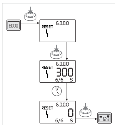
Rys. 53: Potwierdzenie błędu typu B ( X = Y )
