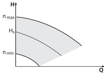
Fig. 46: Varvtalsstyrning
