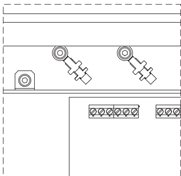
Fig. 26: Kabelavskärmning
