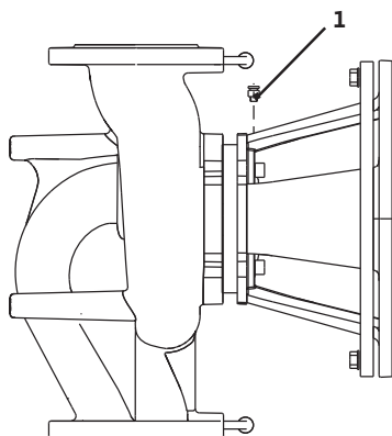
Rys. 43: Zawór odpowietrzający
