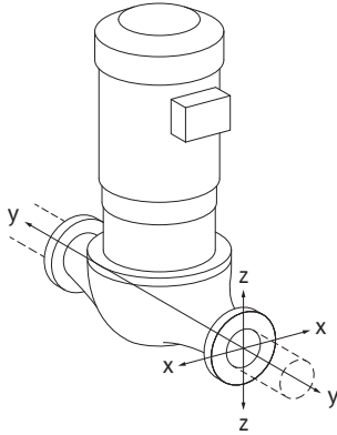
Kuva 22: Kuormitustapaus 16A
