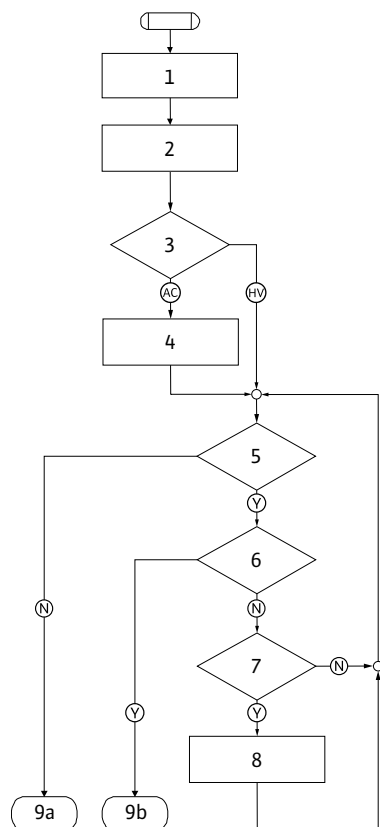
Rys. 56: Typ błędu E, schemat
