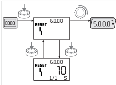
Fig. 47: Fel navigering
