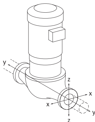
Fig. 22: Расчетный случай нагрузки 16A
