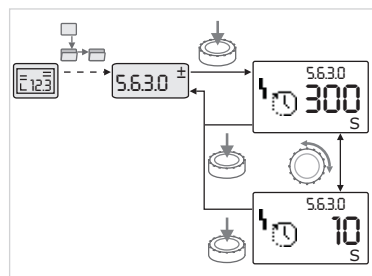
Fig. 40: Inställning med återgång till menyelementet "Val/inställningar"
