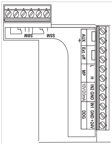
Rys. 27: Zaciski sterujące
