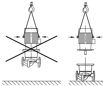
Рис. 8: Транспортировка электродвигателя
