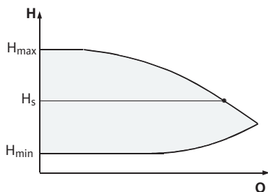
Kuva 10: Säätö \Delta p-c
