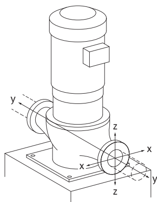
Rys. 23: Przypadek obciążenia 17A
