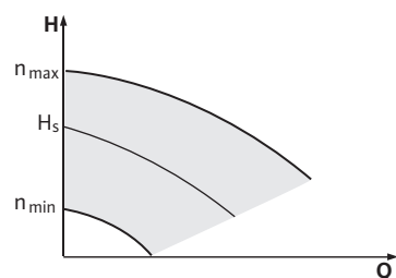
Rys. 46: Tryb sterowania
