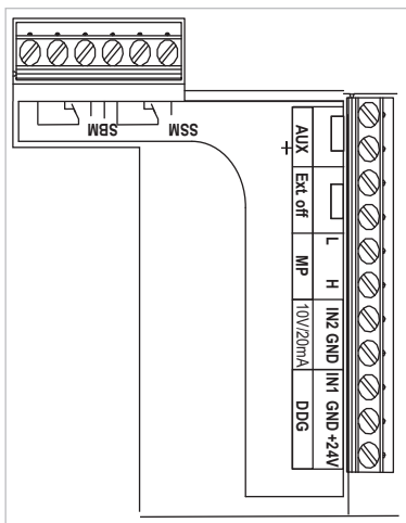
Рис. 27: Клеммы управления
