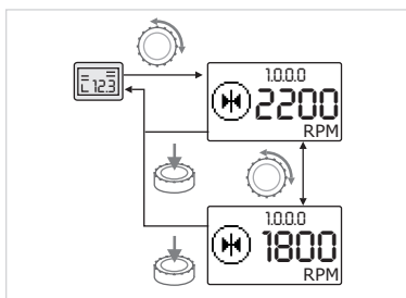
Fig. 35: Inmatning av börvärde
