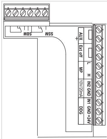
Kuva 27: Ohjausliittimet
