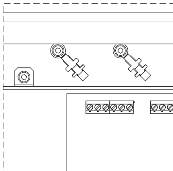
Рис. 26: Экранирование кабелей
