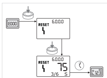
Рис. 52: Квитирование ошибки типа В (X < Y)
