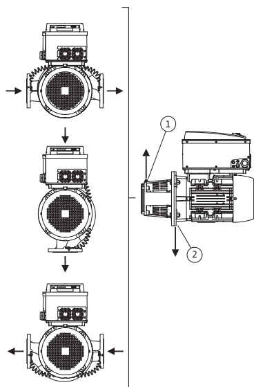
Rys. 18: Dopuszczalne pozycje montażowe z poziomym wałem silnika
