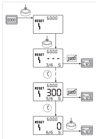
Rys. 55: Potwierdzenie błędu typu C
