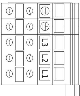
Rys. 28: Zaciski mocy (zaciski sieciowe)
