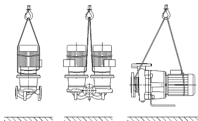
Kuva 7: Pumpun kuljetus
