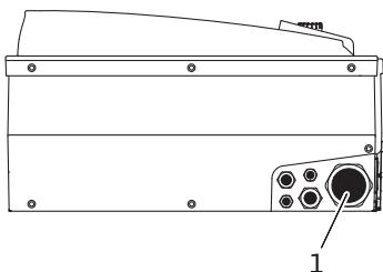
Kuva 25: Kaapelin kierreläpivienni M25/M40
