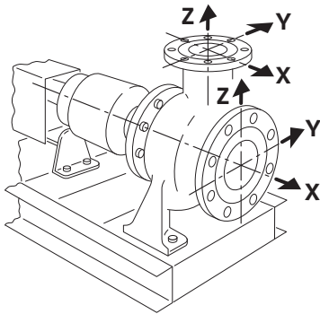
Fig. 24: Lastfall 1A
