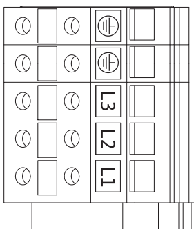
Kuva 28: Teholiittimet (verkkoliittimet)
