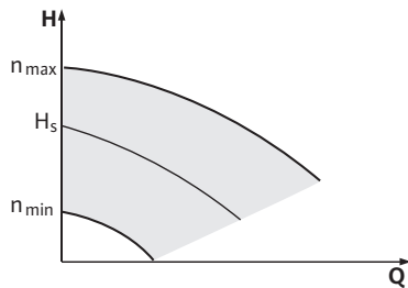
Fig. 12: Varvtalsstyrning
