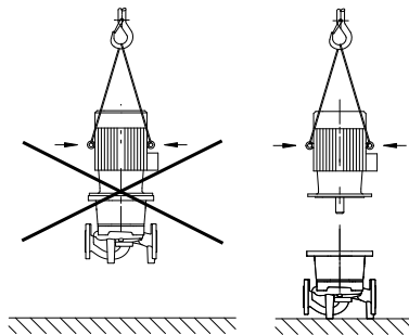
Rys. 20: Transport silnika
