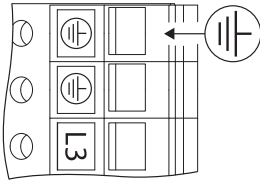
Kuva 29: Lisämaadoitus
