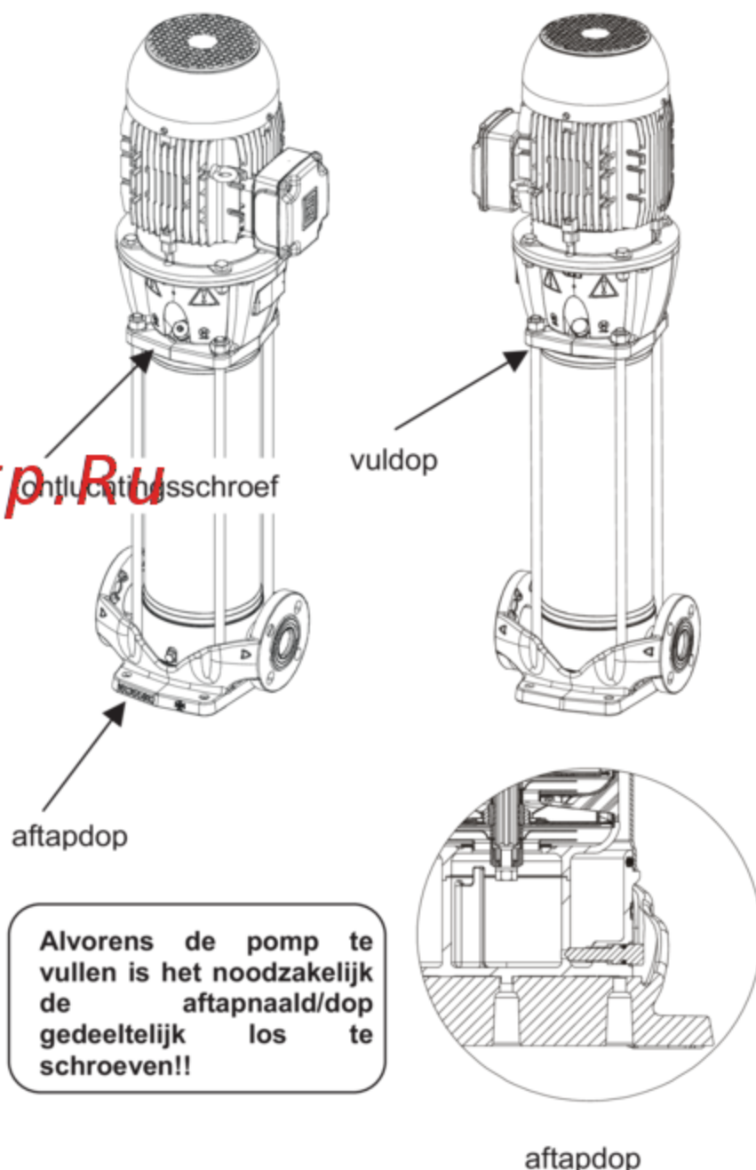
Afb. 6 NKV
