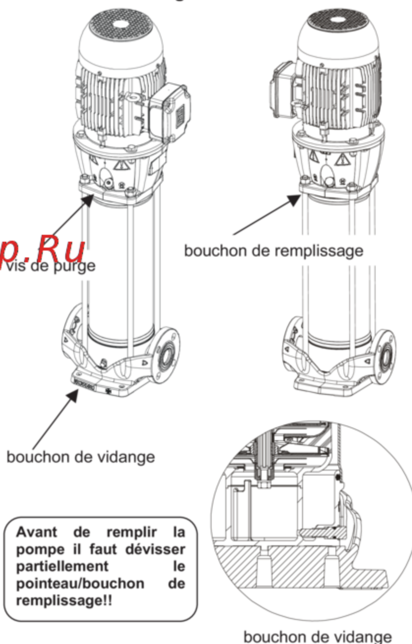
Fig. 6 NKV
