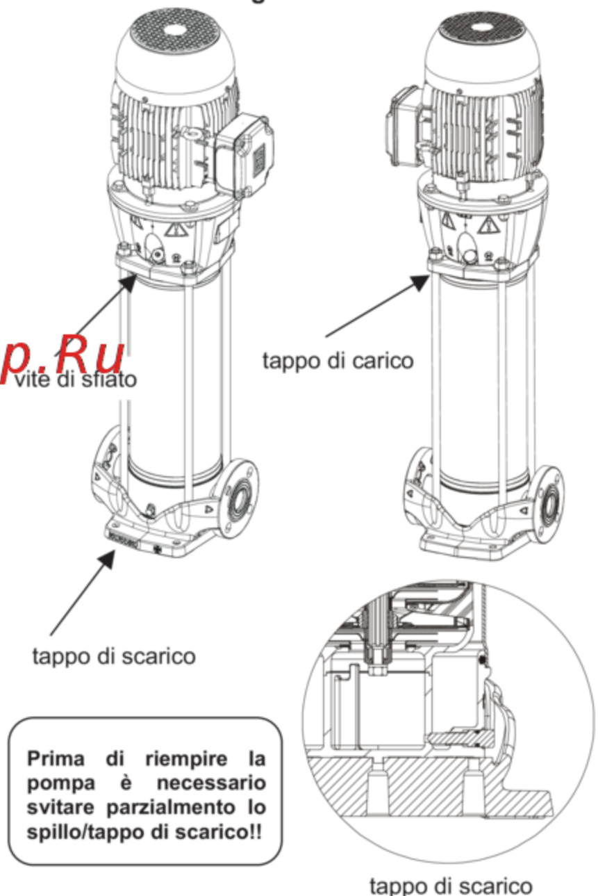
Fig. 6 NKV
