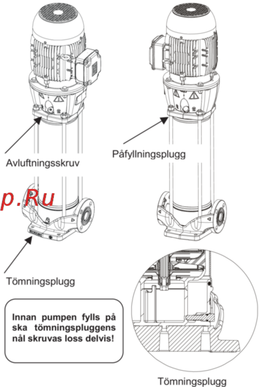
Fig. 6 NKV
