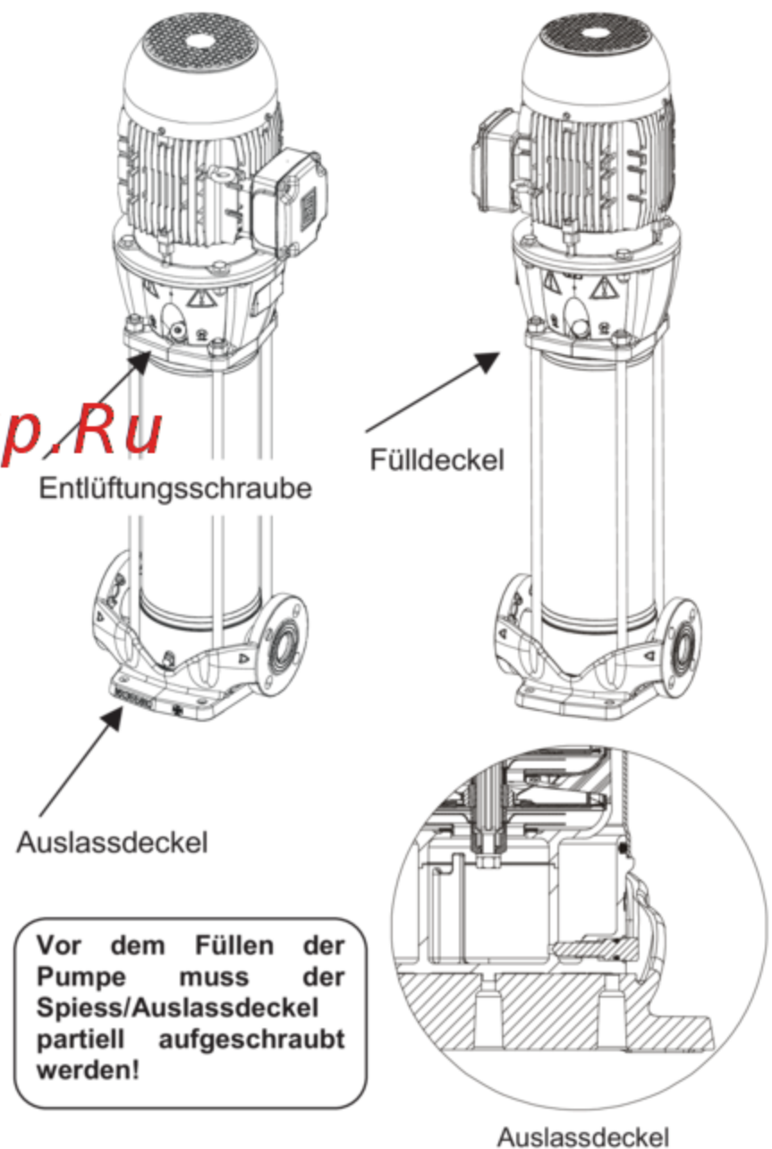
Abb. 6 NKV
