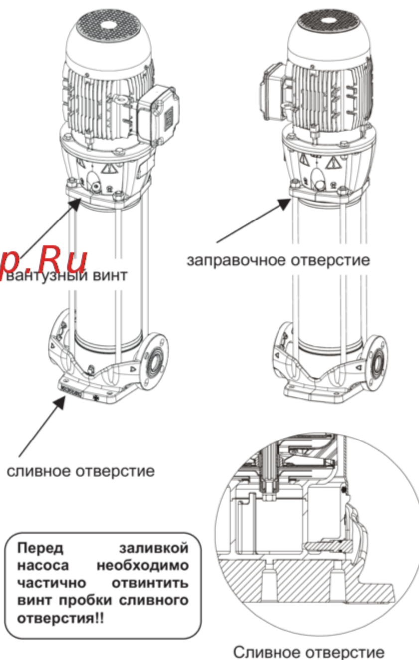
Рис. 6 NKV
