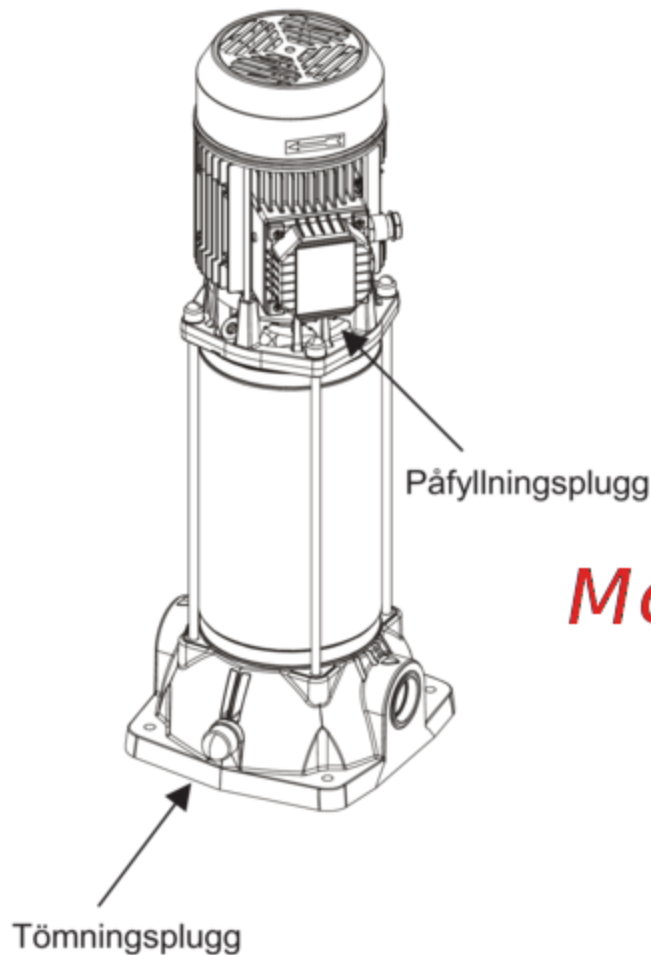
Fig. 5 KVC - KVCX
