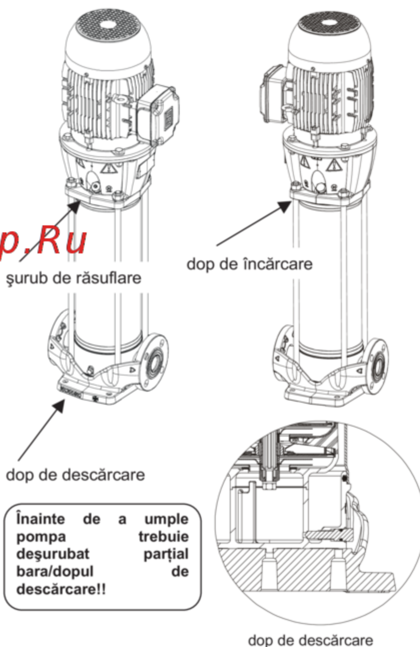
Fig. 6 NKV
