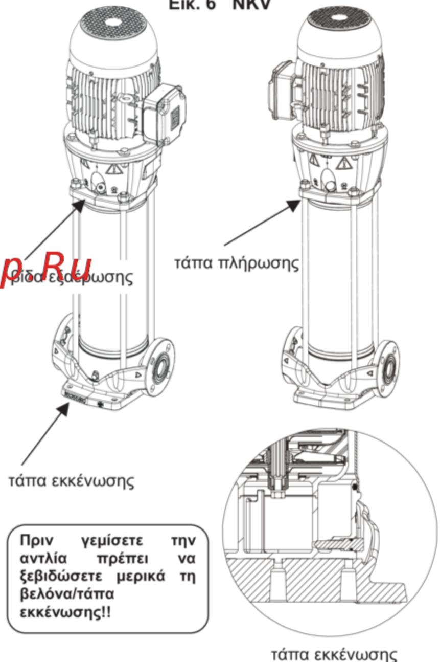
Εικ. 6 NKV
