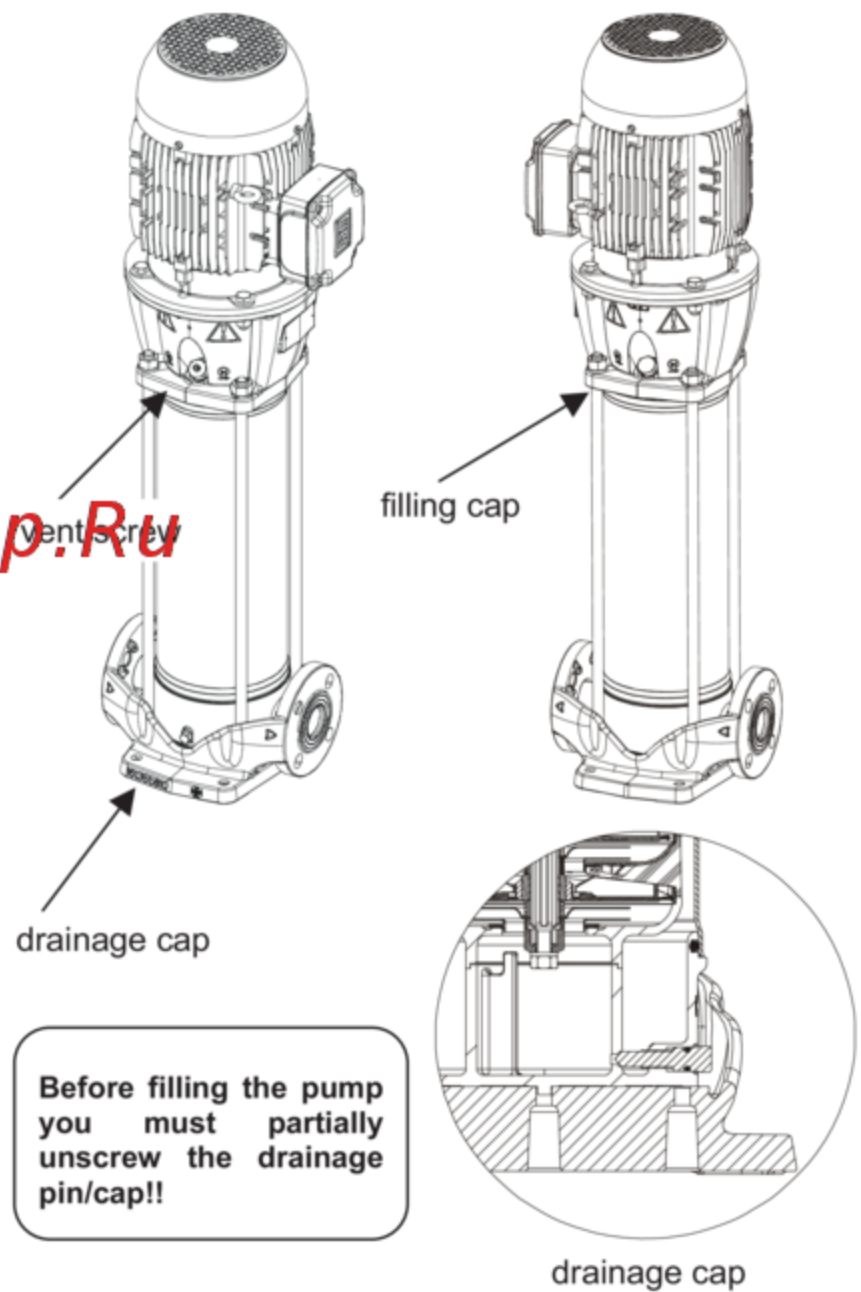
Fig. 6 NKV
