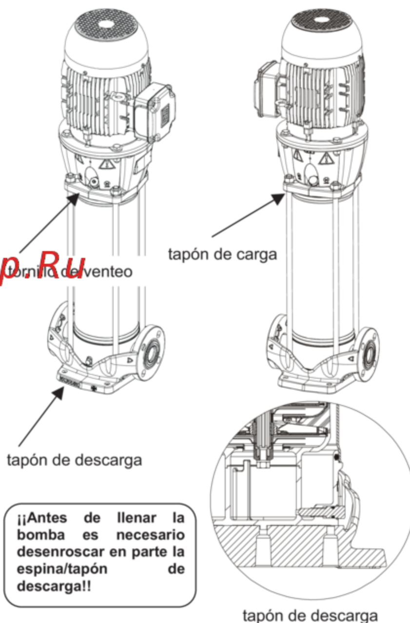
Fig. 6 NKV
