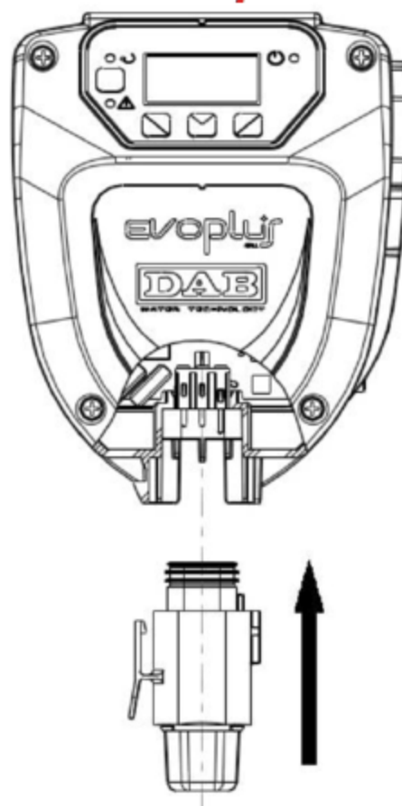
Сх. 3: Каблурованне сетевогa разъема
