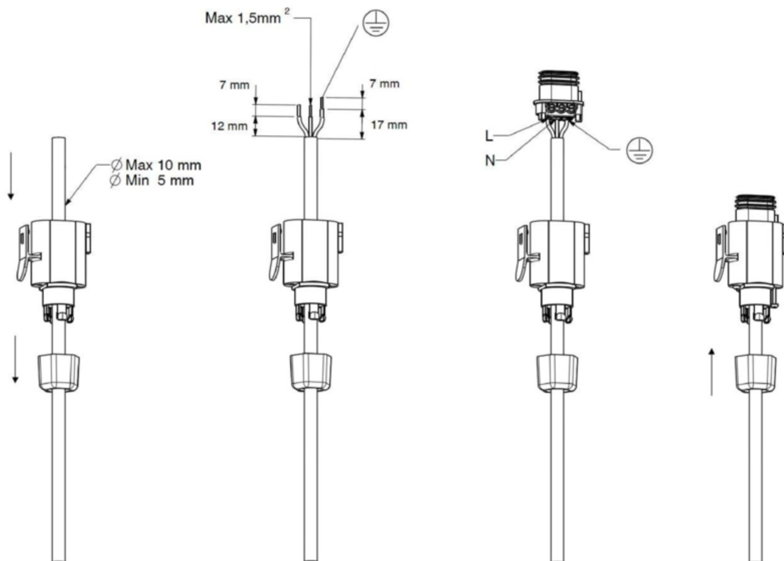
Сх. 3: Каблурованне сетевогa разъема
